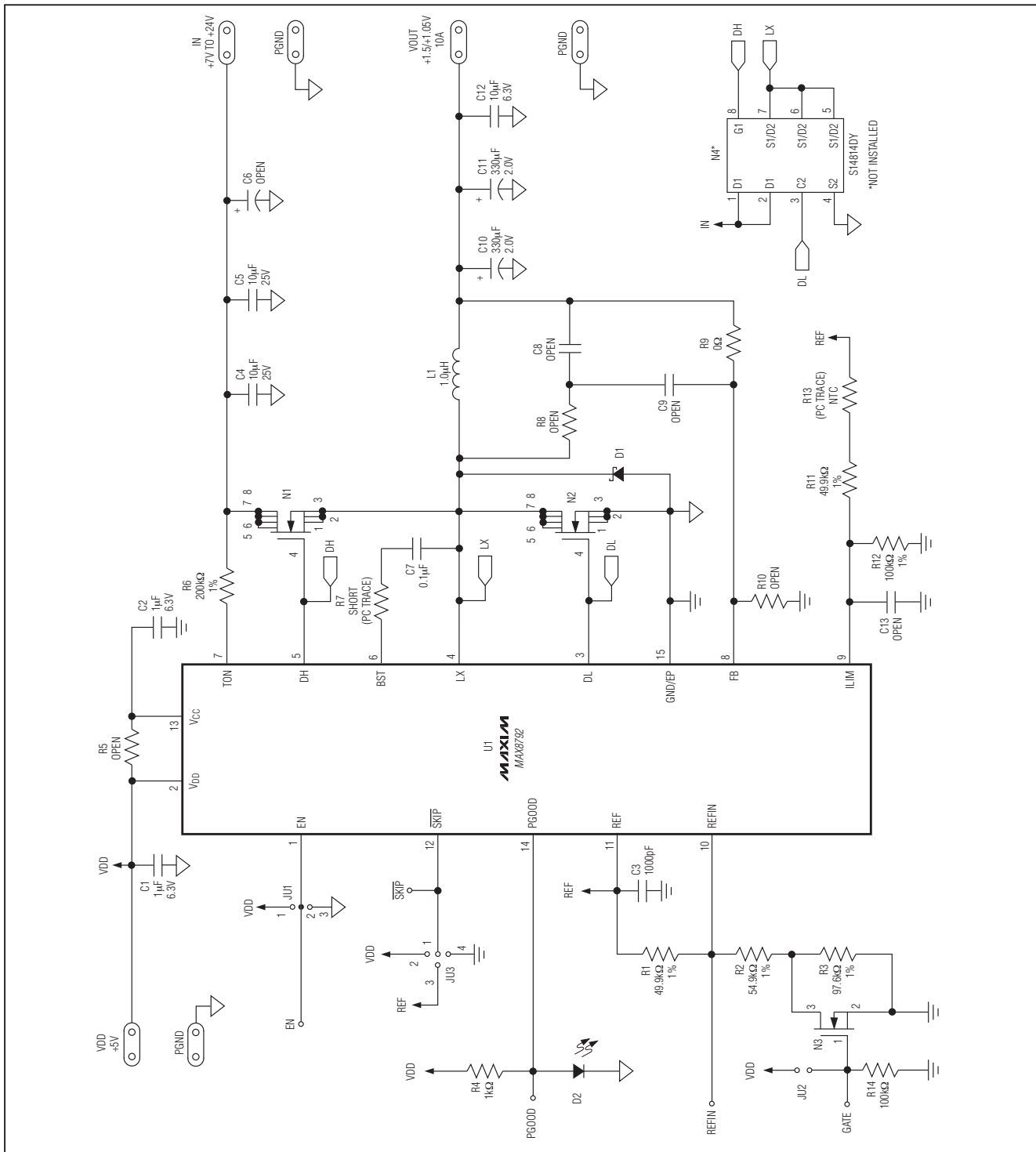
図1. MAX8792のEVキットの回路図
