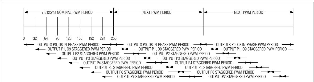
図3. スタッガされたPWM波形
