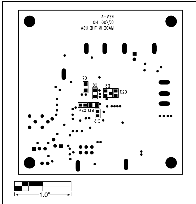
図5. MAX1772EVキットの部品配置図(ハンダ面側)
