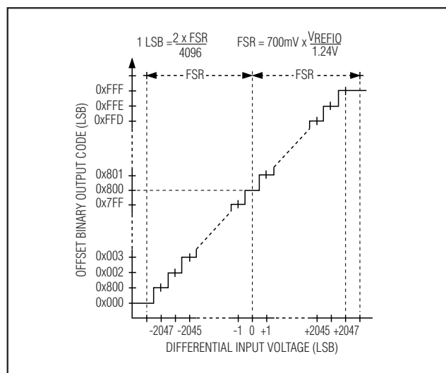
図7. バイナリの伝達関数( \bar{T}/B = 1 )
