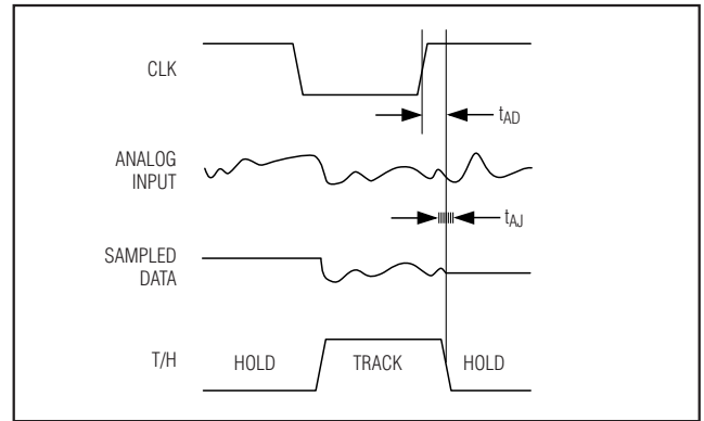
図11. アパーチャジッタ/遅延の仕様
