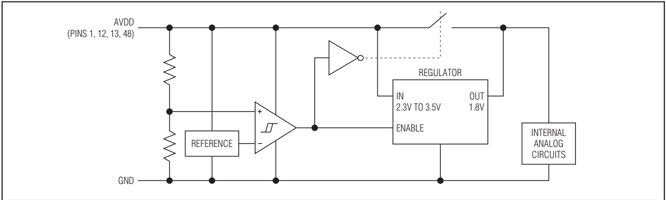
图17. 内部稳压器
