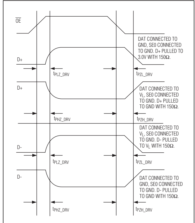
图5. 发送器使能和禁止时序
