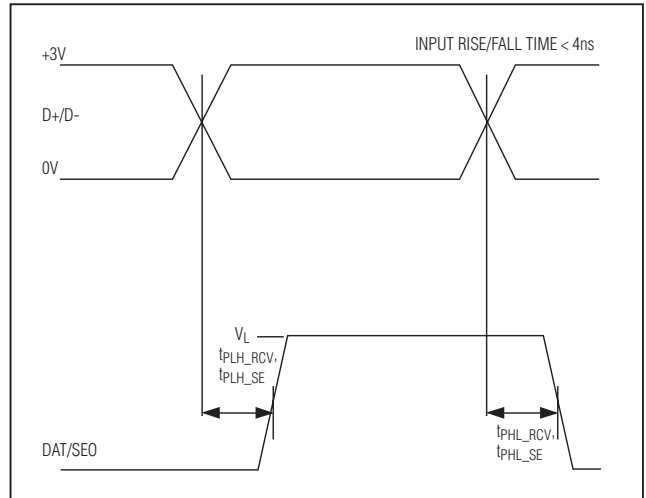
图6. D+/D-相对DAT、SE0的传输延时
