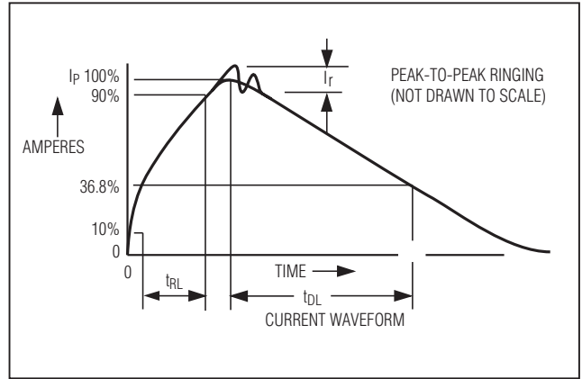
图12. 人体ESD测试模型电流波形
