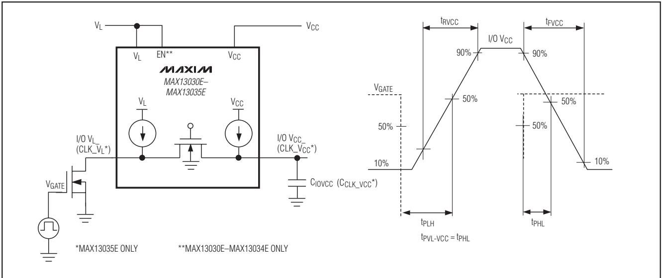
图2. 漏极开路驱动 V_L 侧 I/O 的测试电路和时序
